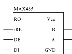
图 3 MAX485 芯片引脚
