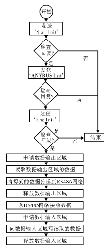
图 5 系统软件框图
