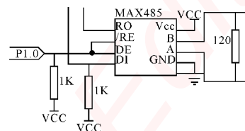
图 4 RS485 接口电路
